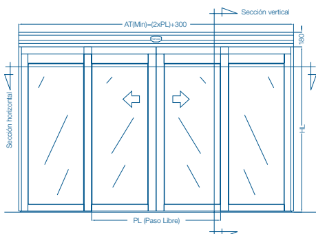
Sección horizontal
