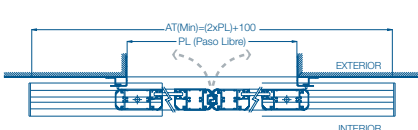
Sección horizontal
