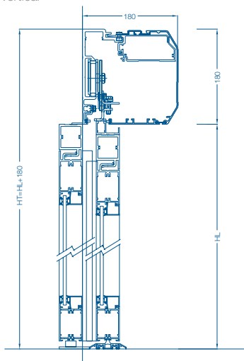
Sección vertical
