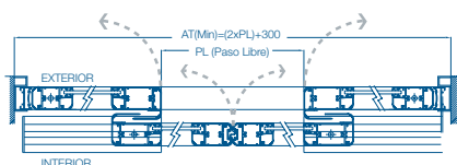
Sección horizontal
